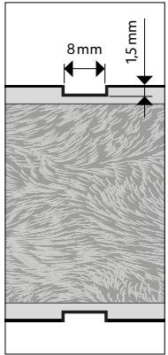
Detail drážky dveří Siluet
