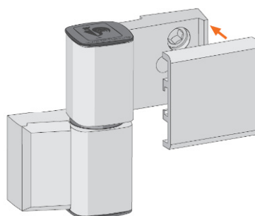
Nasunutí krytky
