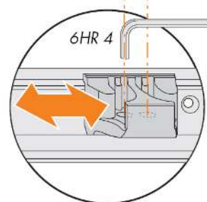
Seřízení koncového dorazu
