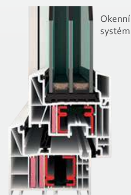
termická výztuha
