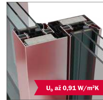
PRŮŘEZ KŘÍDLY SLIM
